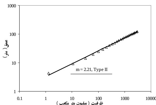
شکل ۱۲. مقدار m و تیپ مخزن سد شهید عباسپور در
