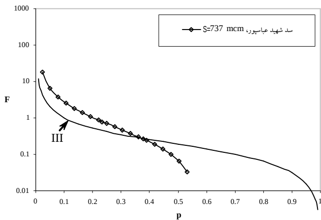
شکل ۶. منحنی مشخص کننده عمق نسبی رسوب برای سد شهید عباسپور
