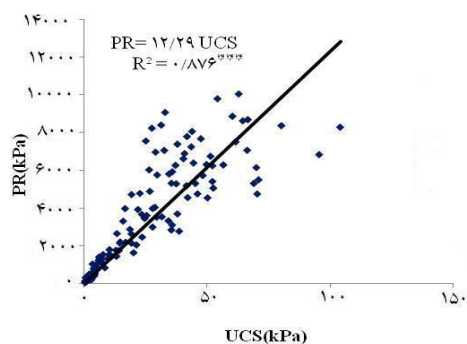
شکل ۴. مقادیر مقاومت فروروی (PR) در برابر مقاومت فشاری غیرمحصور (UCS) برای خاک‌های مورد بررسی
