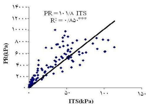
شکل ۳. مقادیر مقاومت فروروی (PR) در برابر مقاومت کششی (ITS) برای خاک‌های مورد بررسی
