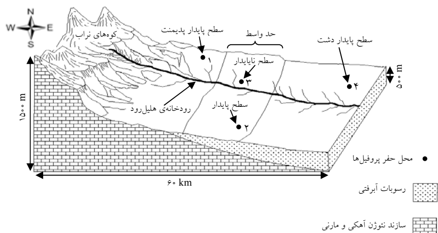
شکل ۲. موقعیت خاک‌های شاهد در سطوح ژئومرفیک انتخاب‌شده
