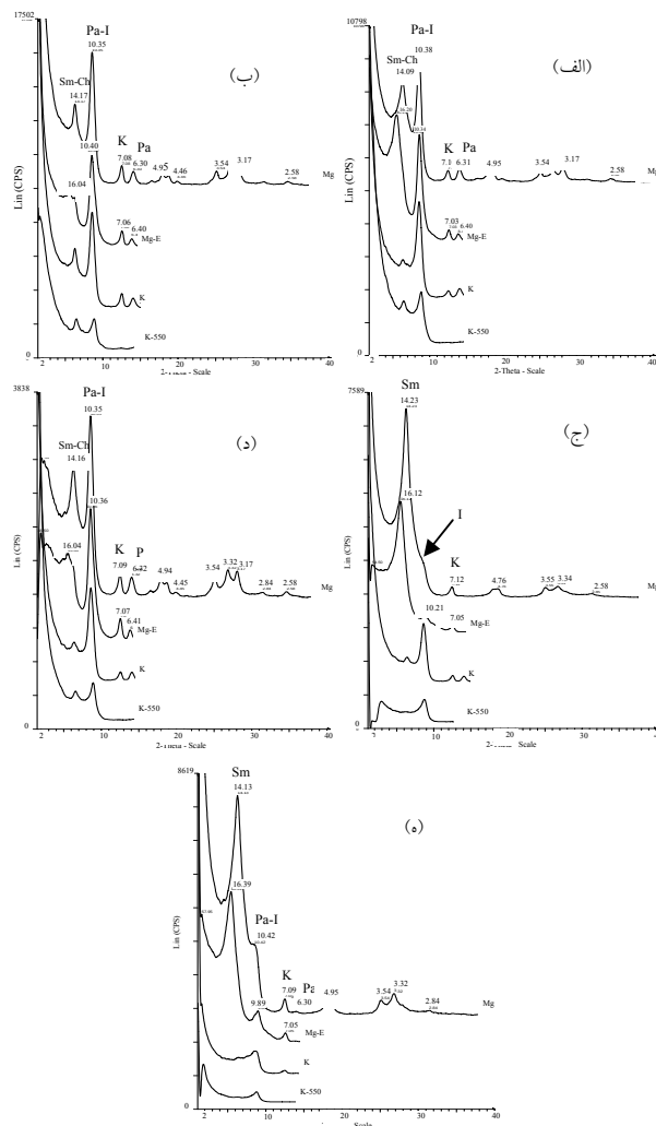
شکل ۴. الف) نمودارهای پراش پرتو ایکس در افق Btk خاکر اول، ب) افق Btk1 خاکر دوم، ج) افق Btn1 خاکر سوم، د) افق 2Btk خاکر سوم، ه) افق Btk2 خاکر چهارم (Mg): اشباع با منیزیم، Mg-E: اشباع با منیزیم و اتیلن گلیکول، K: اشباع با پتاسیم، K-550: اشباع با پتاسیم و حرارت ۵۵۰ درجه سانتی گراد؛ Sm: اسمکتیت، I: ایلیت، K: کانولینیت، Pa: پالیگورسکیت، Ch: کلریت
