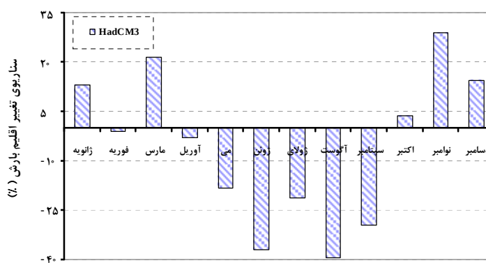
شکل ۶. سناریوهای تغییر اقلیم بارندگی از مدل HadCM3
