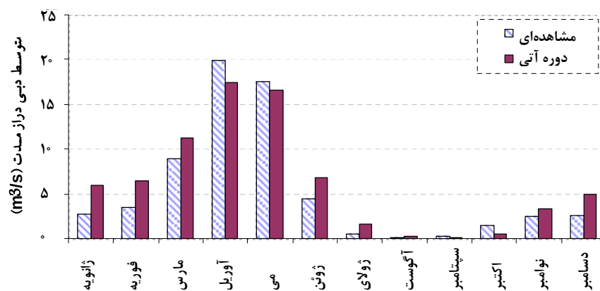
شکل ۹. مقایسه میانگین دراز مدت ماهانه رواناب دوره آتی و دوره مشاهداتی
