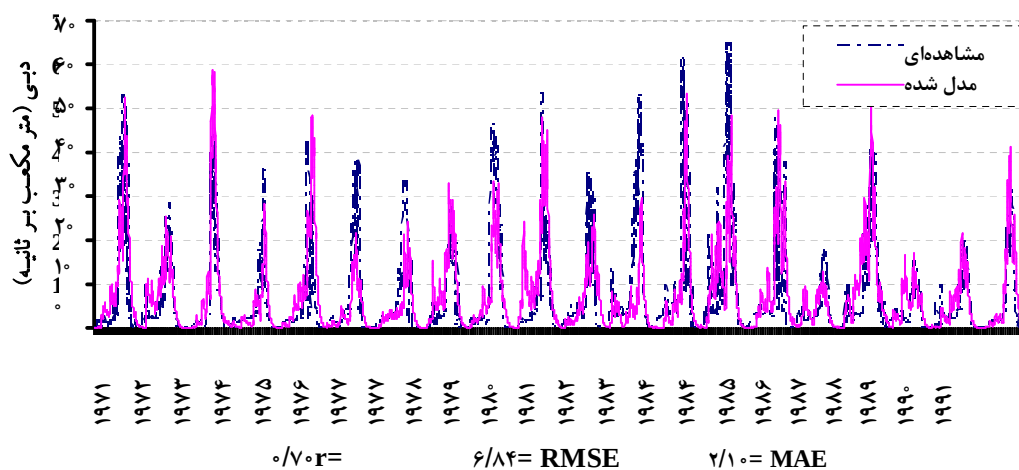
شکل ۸. مقایسه رواناب مشاهداتی حوضه آیدوغموش با رواناب مدل شده در دوره صحت‌یابی ۱۹۷۱ - ۱۹۹۱
