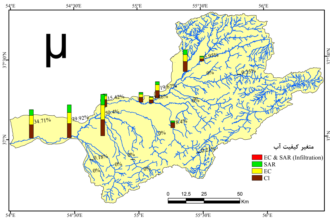
شکل ۶. فراوانی تجاوز متغیرهای کیفیت آب از استاندارد کیفیت آب کشاورزی در حوضه گرگانرود (اعداد نشان دهنده درصد آزمایش های مرود برای هر ایستگاه هیدرومتری و رنگها نشان دهنده درصد موارد تجاوز از استاندارد برای هر متغیر کیفیت آب است)
