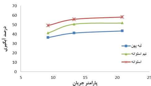
شکل ۹. تغییرات میزان آبگیری سرریزهای جانبی با ارتفاع ۱۲۵ میلی‌متر با بازشدگی ۱۰ سانتی‌متر در دریچه انتهایی
