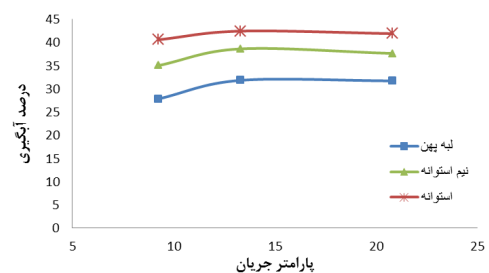
شکل ۱۰. تغییرات میزان آبگیری سرریزهای جانبی با ارتفاع ۱۲۵ میلی‌متر با باز شدگی ۵ سانتی‌متر در دریچه انتهایی
