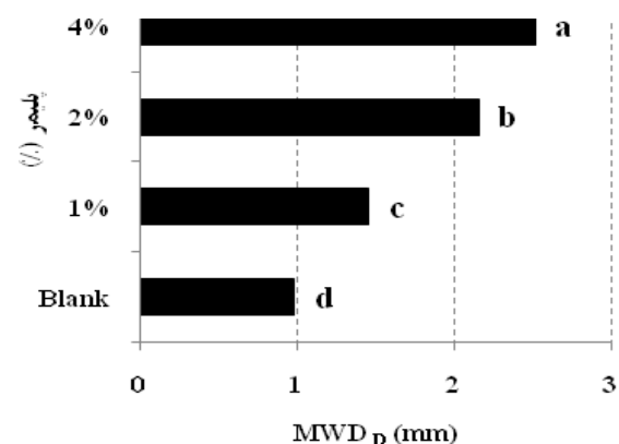
شکل ۷. تأثیر غلظت پلیمر پلی‌الکترولیت آنیونی بر MWDD (میانگین‌های دارای حروف مشابه در سطح ۵ درصد آزمون دانکن فاقد اختلاف معنی دار می‌باشند)
