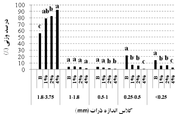
شکل ۸. کلاس توزیع اندازه ذرات با درصدهای متفاوت پلیمر (میانگین‌های دارای حروف مشابه در سطح ۵ درصد آزمون دانکن فاقد اختلاف معنی دار می‌باشند)
