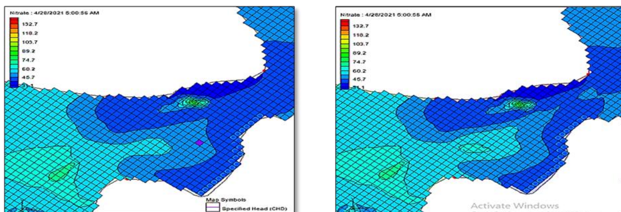
شکل ۱۰. تأثیر کیفی رهاسازی پساب در رودخانه بر کیفیت آبخوان در سال ۱۴۰۰ نسبت به شرایط بدون تغذیه
