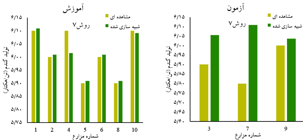
شکل ۴. شبیه سازی تولید گندم با استفاده از شاخص های گیاهی تحت روش های مختلف و به کارگیری روش رگرسیون بردار پشتیبان (ادامه)
