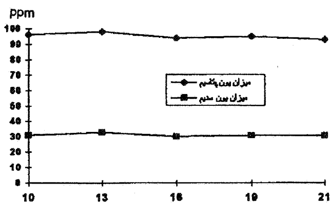
شکل ۳. تغییر غلظت الکترولیت‌ها در رقم تلقیح نشده و پایدار ILC ۵۹۲۸
