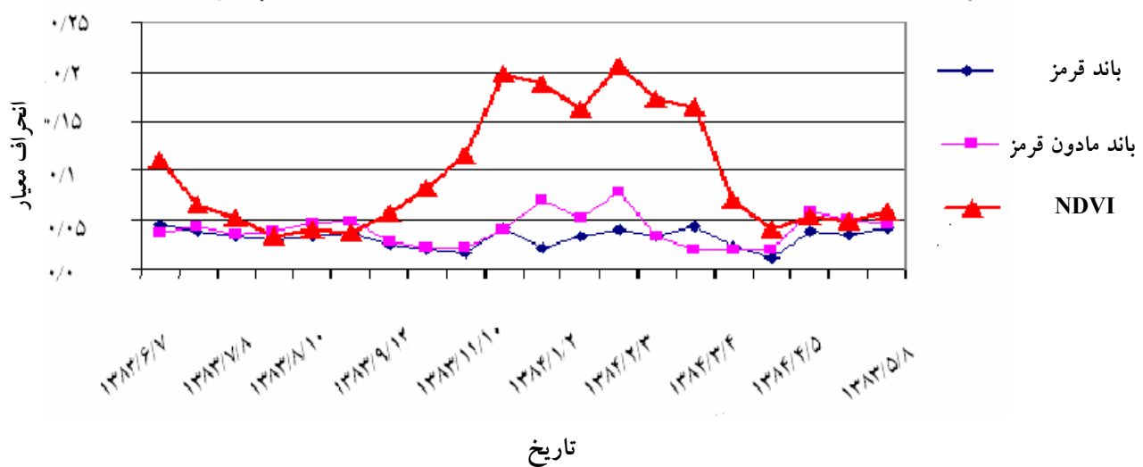
شکل ۳. تغییرات انحراف معیار بانده قرمز، مادون قرمز و شاخص NDVI در ۴ مزرعه گندم واقع در حومه مشهد (محدوده مزرعه نمونه آستان قدس رضوی) در سال زراعی ۸۴-۸۳
