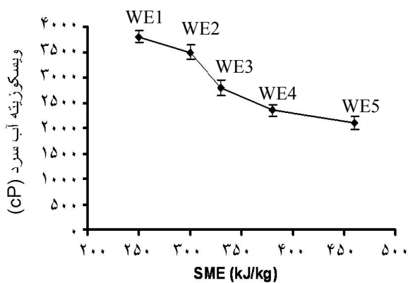
شکل ۱۱. نمودار ویسکوزیته آب سرد (در دمای ۲۵ °C) به دست آمده از دستگاه RVA نمونه‌های اکستروژن شده با SME های متفاوت
