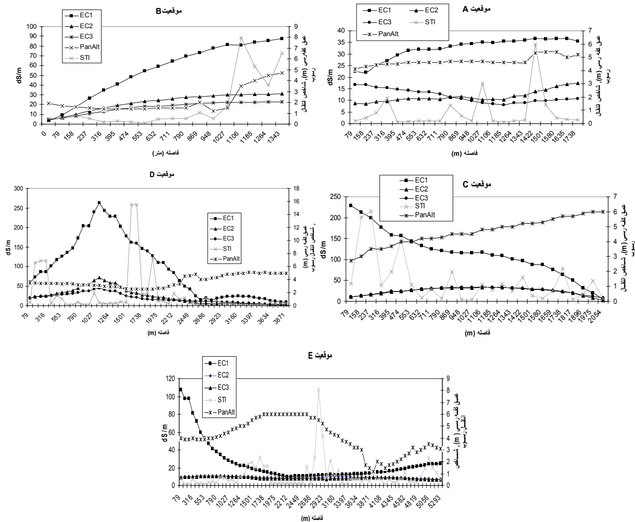
شکل ۸. نمودارهای ترانسکت‌ها در موقعیت‌های A، B، C، D و E و رابطه آنها با شوری ۵۰-۱۰۰ سانتی‌متر (EC1)، ۱۰۰-۱۵۰ سانتی‌متری خاک (EC2) (دسی زیمنس بر متر)، شاخص انتقال رسوب (STI) و عمق کفه رسی (PanAlt).
