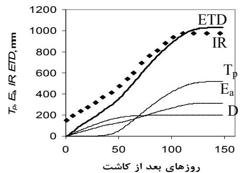
شکل ۵. مقادیر پیش‌بینی شده نفوذ عمقی (D)، تبخیر از سطح خاک (Ea)، تعرق بالقوه (Tp)، مجموع تبخیر، تعرق و نفوذ عمقی (ETD) توسط مدل MSM و مقادیر اندازه‌گیری شده آب آبیاری و بارندگی (IR) در سال ۱۳۸۳
