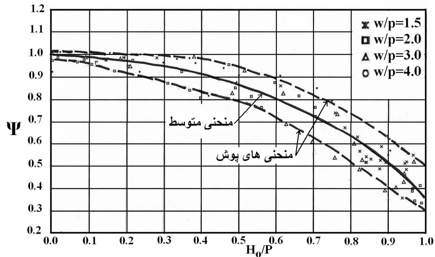
شکل ۷. ضریب تصحیح استغراق جریان ( \psi ) به صورت تابعی از h_d/h به ازای (R/w = 0/15) - آزمون (W3-Ri)
