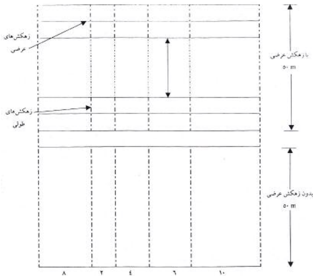
شکل ۱. کروکی تیمارهای با زهکش عرضی و بدون زهکش عرضی و ابعاد آنها (بر حسب متر) در یک تکرار
