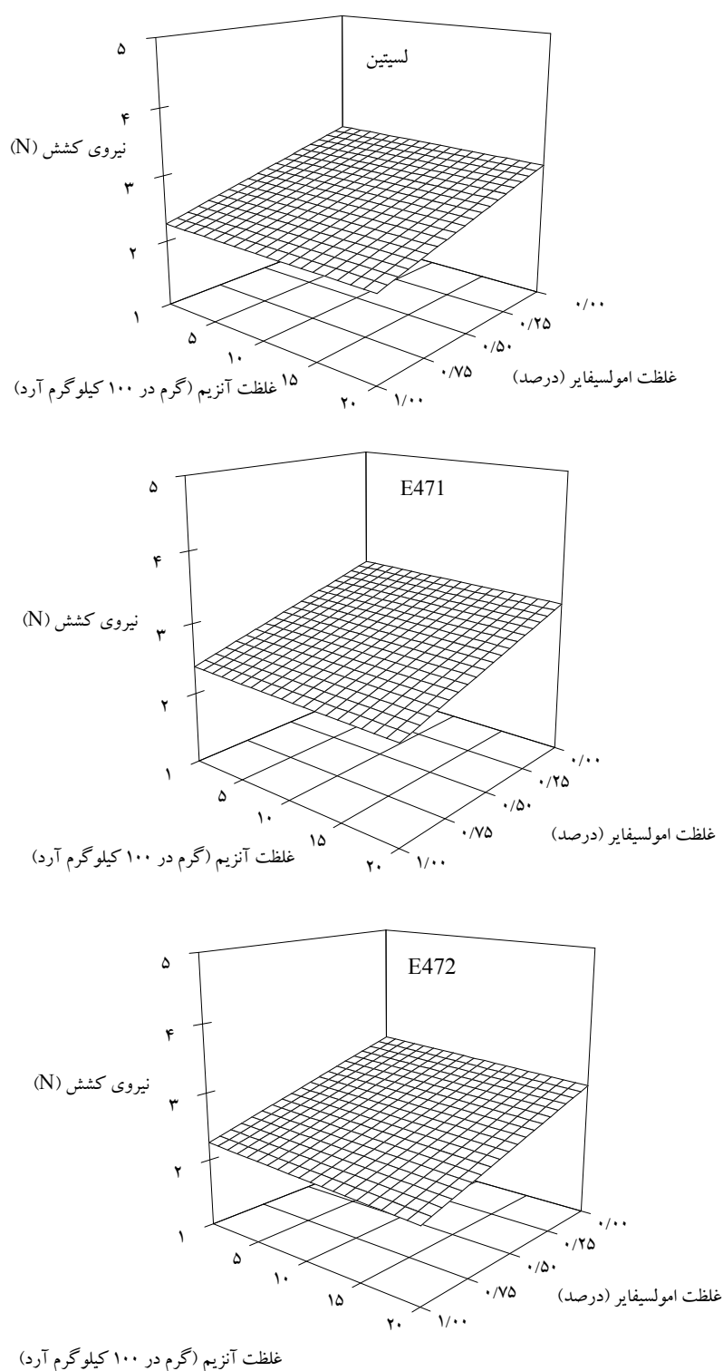
شکل ۵. نیروی کشش نان بر حسب غلظت امولسیفایرهای لستین، E471، E472 و آنزیم \alpha -آمیلاز در زمان تولید که از طریق تجزیه سطح عکس العمل برازش شده است.
