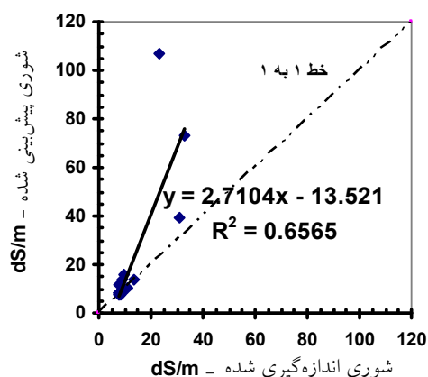
شکل ۳. مقایسه مقادیر اندازه‌گیری شده شوری در برابر مقادیر پیش‌بینی شده با مدل SWAP (بالاچپ) LEACHC (بالا راست) و معادله ۱ (پایین) در تیمار DIL1
