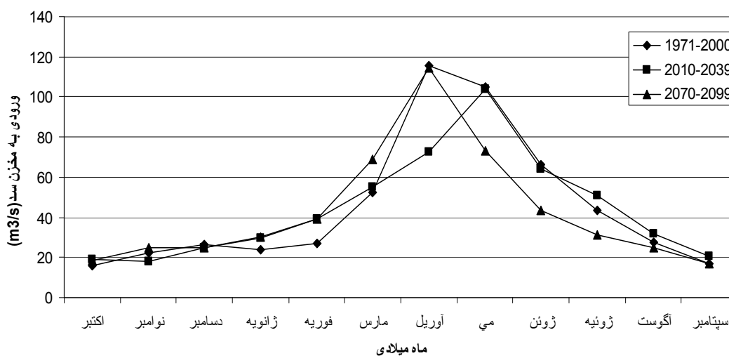
شکل ۶. میانگین متوسط ماهانه دراز مدت دبی ورودی به مخزن، طی دوره مشاهده شده و دوره‌های تغییرات اقلیمی سناریوی A2
