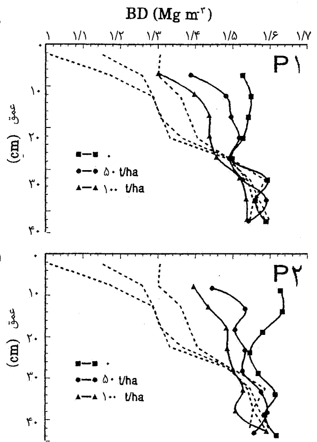
شکل ۳- تأثیر سطوح مختلف کودی در رطوبت PL با یک عبور (P ۱ ) و دو عبور (P ۲ ) تراکتور بر BD و مقایسه نظیر به نظیر آنها با شاهدهای مربوطه (منحنیهای خط چین)
