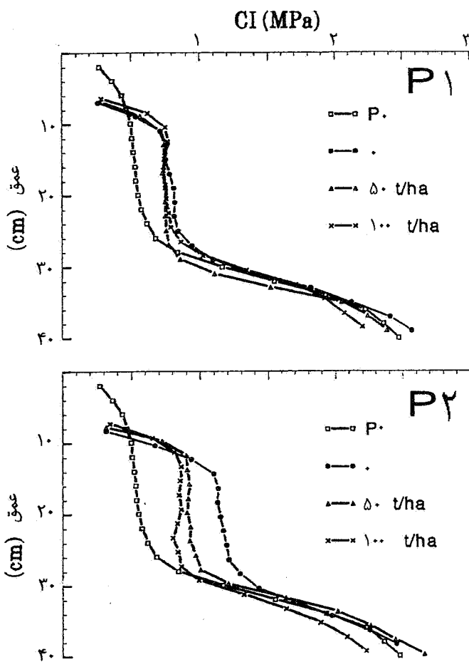
شکل ۴- تأثیر سطوح مختلف کودی در رطوبت PL با یک عبور (P ۱ ) و دو عبور (P ۲ ) تراکتور بر CI و مقایسه نظیر به نظیر آنها با شاهدهای مربوطه (منحنیهای خط چین)
