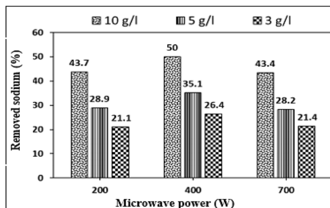
شکل ۹. میانگین نتایج حذف سدیم توسط نانوجاذب فعال مغناطیسی تحت اثر میدان مغناطیسی به ازای توان یکسان ماکروویو
