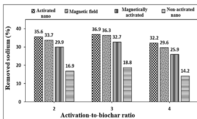
شکل ۱۵. تأثیر نسبت فعالساز در حذف یون سدیم توسط جاذبها
