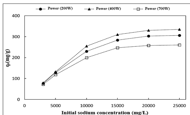
شکل ۲۲. تأثیر غلظت اولیه یون سدیم در مقدار حذف توسط نانوجاذب فعال مغناطیسی تحت اثر میدان مغناطیسی
