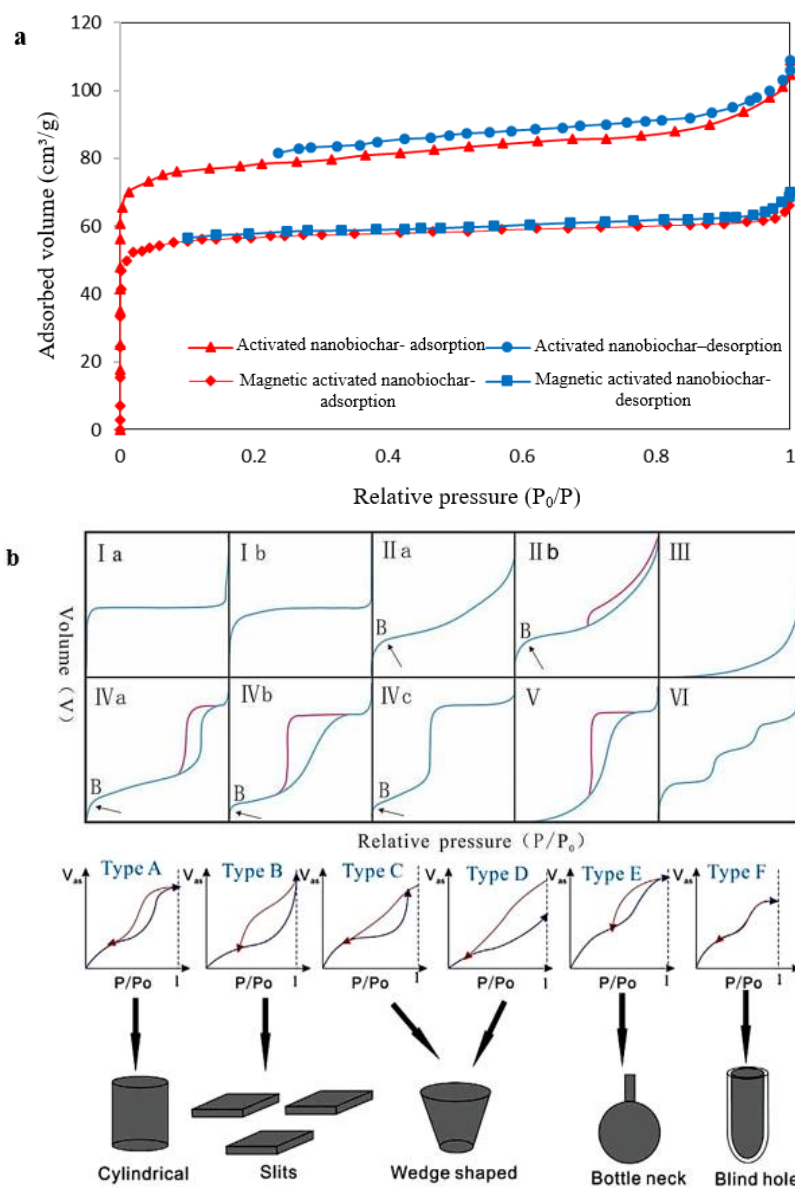
شکل ۵. (a) نتایج جذب و واجذب نیتروژن، (b) تصویر انواع استاندارد ایزوترم‌های جذب به همراه انواع شکل منافذ
