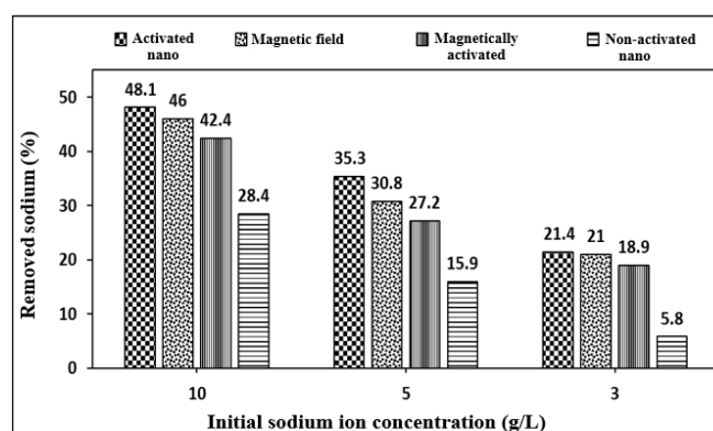
شکل ۱۶. تأثیر غلظت اولیه در حذف یون سدیم توسط جاذبها
