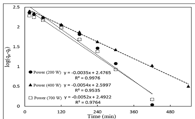
شکل ۱۸. برازش مدل سینتیکی شبه مرتبه اول بر نتایج اندازه‌گیری شده حذف سدیم در نانوجاذب‌های فعال مغناطیسی تحت اثر میدان مغناطیسی
