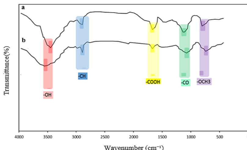
شکل ۳. (a) طیف سنجی نانو جاذب فعال قبل از حذف، (b) طیف سنجی نانو جاذب فعال بعد از حذف \text{Na}^+
