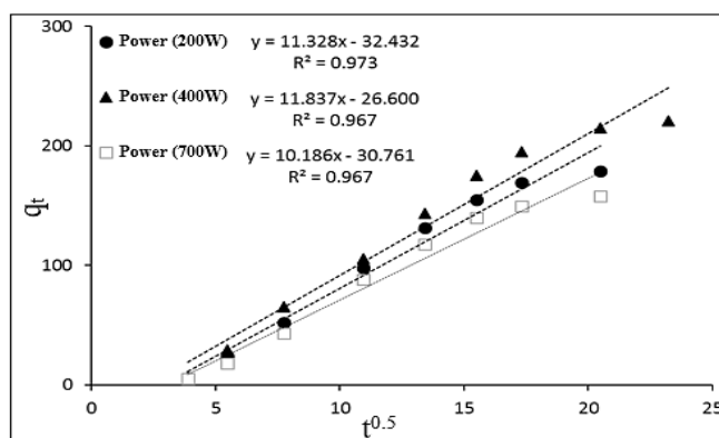
شکل ۲۱. برازش مدل سینتیکی نفوذ درون ذره‌ای بر مقادیر آزمایشگاهی حذف یون سدیم توسط نانوجاذب فعال مغناطیسی تحت اثر میدان مغناطیسی
