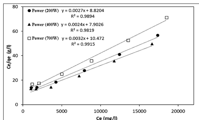
شکل ۲۳. برازش مدل هم‌دمای جذب لانگمویر بر مقادیر اندازه‌گیری شده یون سدیم توسط نانوجاذب‌های فعال مغناطیسی تحت اثر میدان مغناطیسی
