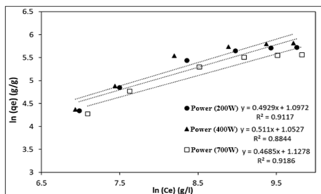
شکل ۲۴. برازش مدل فروندلیچ بر مقادیر حذف سدیم توسط نانوجاذب‌های فعال مغناطیسی تحت اثر میدان مغناطیسی
