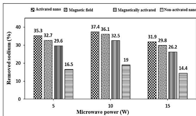
شکل ۱۴. تأثیر زمان فعالسازی در حذف یون سدیم توسط جاذب
