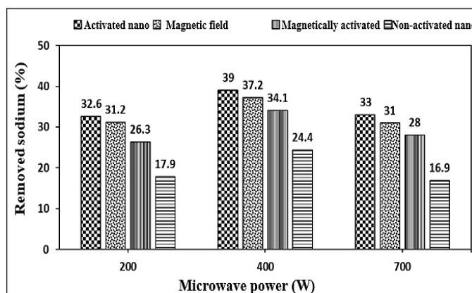
شکل ۱۳. تاثیر توان ماکروویو در حذف یون سدیم توسط جاذب‌ها
