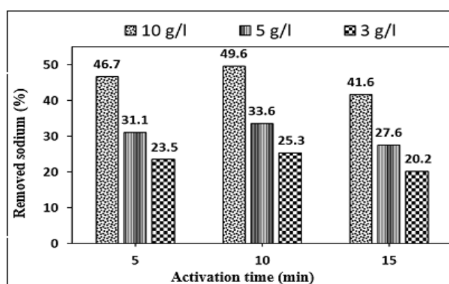
شکل ۱۰. میانگین نتایج حذف یون سدیم توسط نانوجاذب فعال مغناطیسی تحت اثر میدان به ازای مدت فعالسازی یکسان
