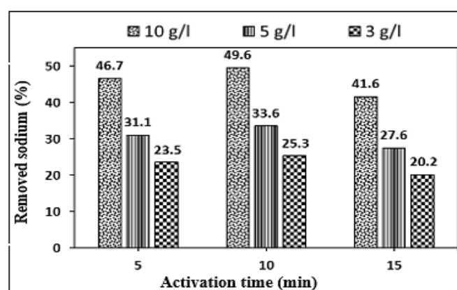
شکل ۱۱. میانگین نتایج حذف سدیم توسط نانوجاذب فعال مغناطیسی تحت اثر میدان به ازای نسبت فعالساز یکسان
