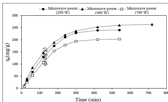
شکل ۱۷. تأثیر مدت زمان تماس در مقدار حذف یون سدیم توسط نانو زغال زیستی فعال مغناطیسی تحت اثر میدان مغناطیسی
