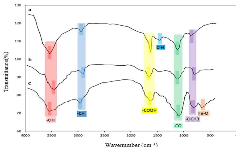
شکل ۲. نتایج طیف سنجی مادون قرمز جاذب‌ها. (a) جاذب غیر نانو فعال، (b) نانو جاذب فعال، (c) نانو جاذب فعال مغناطیسی
