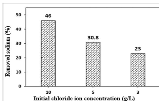
شکل ۱۲. تأثیر غلظت اولیه بر میانگین حذف یون سدیم توسط نانوجاذب فعال مغناطیسی تحت اثر میدان مغناطیسی
