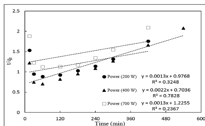
شکل ۱۹. برازش مدل سینتیکی شبه مرتبه دوم بر نتایج اندازه‌گیری شده حذف سدیم در نانوجاذب‌های فعال مغناطیسی تحت اثر میدان مغناطیسی
