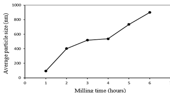
شکل ۱. تاثیر مدت زمان آزمون آسیاب بر اندازه متوسط ذرات
