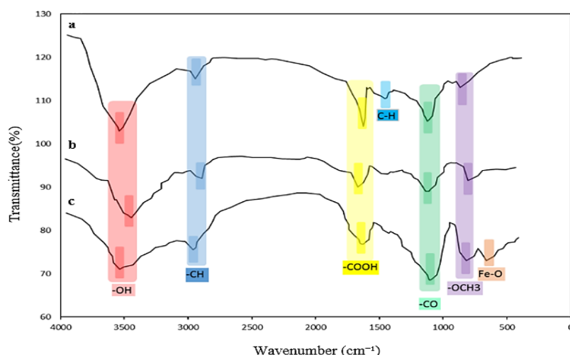
شکل ۲. نتایج طیف سنجی مادون قرمز جاذب‌ها. (a) جاذب غیر نانو فعال، (b) نانو جاذب فعال، (c) نانو جاذب فعال مغناطیسی
