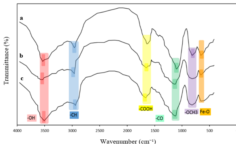
شکل ۴. (a) طیف سنجی نانو بیوچار فعال مغناطیسی قبل از حذف، (b) طیف سنجی نانو بیوچار فعال مغناطیسی بعد از حذف \text{Na}^+
