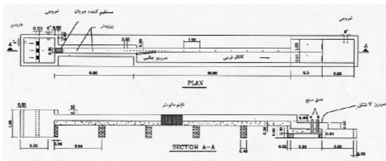
شکل ۱. نمای شماتیک از مدل فیزیکی ساخته شده
