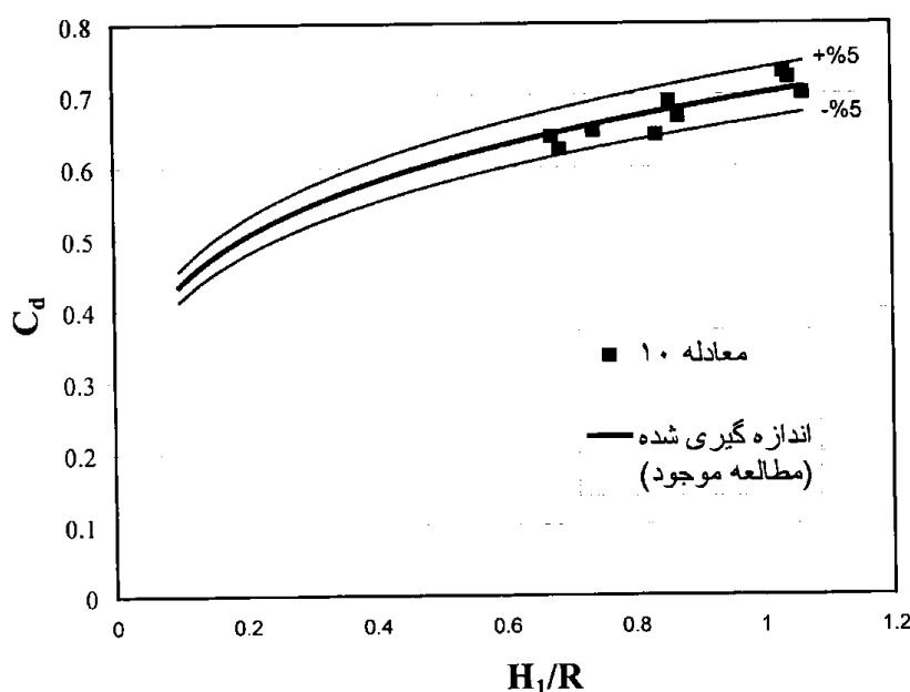
شکل ۱۰. ضریب جریان از طریق اندازه‌گیری مستقیم و معادله ۱۰ برای مدل نیم‌استوانه‌ای با ارتفاعات مختلف
