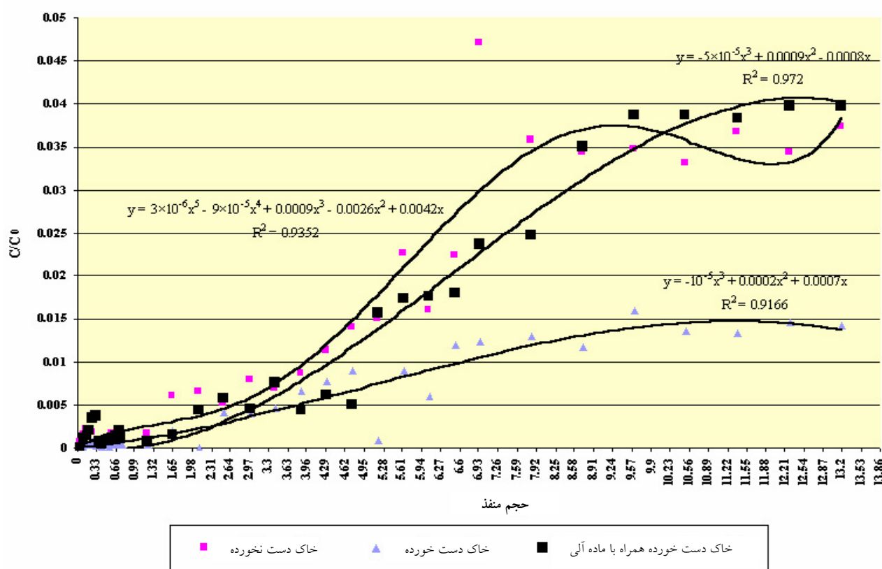
شکل ۳. منحنی‌های انحناي عنصر کادمیوم در حجم منفذها و تیمارهای مختلف خاک
