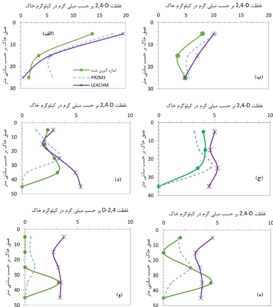
شکل ۱. 2,4-D اندازه‌گیری شده و شبیه‌سازی شده توسط مدل‌های PRZM-3 و LEACHM در اعماق مختلف خاک و در تیمار آبیاری شمال الف) ۸ روز پس از کاربرد، ب) ۱۳ روز بعد از کاربرد، ج) ۲۳ روز بعد از کاربرد، د) ۳۰ روز بعد از کاربرد، ه) ۳۷ روز بعد از کاربرد، و) ۵۷ روز بعد از کاربرد
