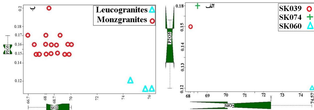
شکل ۳. Binary boxplot SiO 2 vs. P 2 O 5 . الف) سه نمونه سنگ مورد مطالعه و ب) برگرفته از نتایج شبیهی و اسماعیلی (۱)
