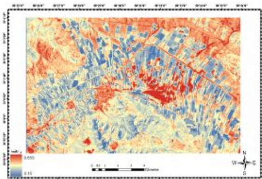
ب) \alpha آلبیدوی سطحی
