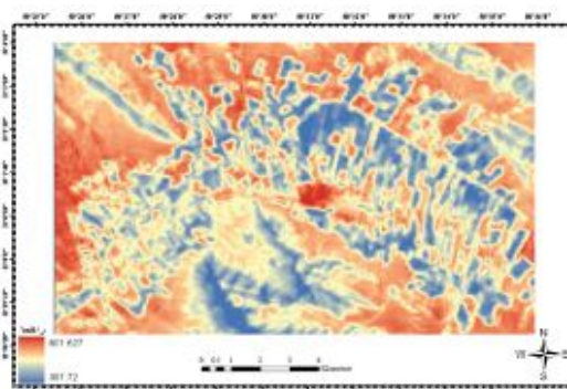
پ) R_{L\downarrow} تابش موج بلند خروجی
