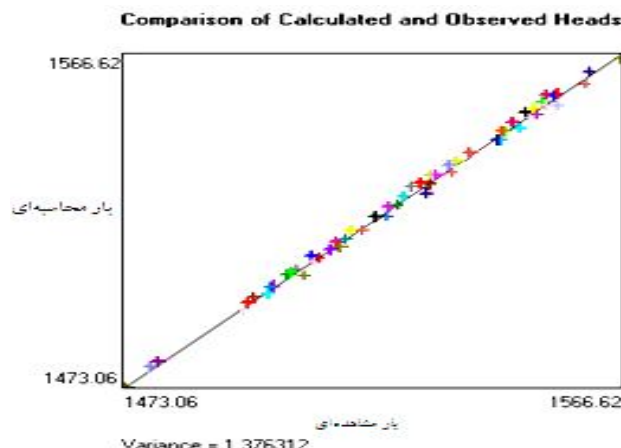
شکل ۸. نتایج تراز هیدرولیکی شبیه‌سازی شده در مقابل مقادیر چاه‌های مشاهده‌ای در حالت ماندگار
