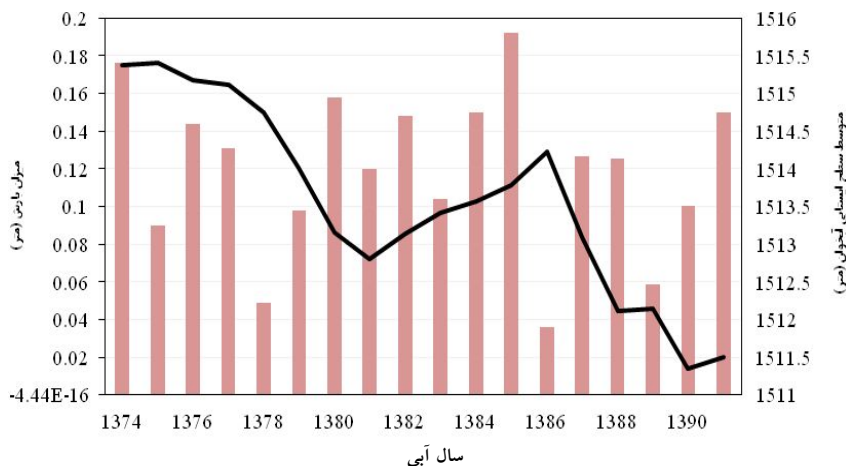
شکل ۷. هیدروگراف آبخیز سطحی زیرحوضه کوهپایه- سگری همراه با بارش سالانه طی سال‌های ۱۳۷۴ تا ۱۳۹۱
