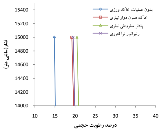
شکل ۱۲. مقایسه منحنی مشخصه خاک بدون عملیات خاک‌ورزی و خاک پادله شده با ادوات خاک‌ورزی مختلف در پژمردگی دائم (۱۵۰۰۰ سانتی متر)
