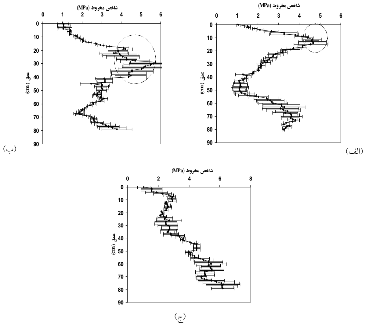
شکل ۶. تغییرات میانگین مقاومت مکانیکی (شاخص مخروط) خاک با عمق برای بافت‌های: الف) لوم شنی با درصد رطوبت وزنی و چگالی ظاهری خاک رویین به ترتیب برابر ۱۲/۴ و ۱/۶۸ مگاگرم بر متر مکعب، ب) لوم رسی با درصد رطوبت وزنی و چگالی ظاهری خاک رویین به ترتیب برابر ۱۵/۹ و ۱/۶۸ مگاگرم بر متر مکعب و ج) رسی با درصد رطوبت وزنی و چگالی ظاهری خاک رویین به ترتیب برابر ۱۵/۴ و ۱/۵۰ مگاگرم بر متر مکعب. مقادیر رطوبت وزنی خاک زیرین به ترتیب برابر ۱۳/۶، ۱۷/۶ و ۱۵/۵ درصد بود. این مزارع تحت بازرویی دوم بودند. میله‌های افقی بیانگر \pm یک خطای معیار می‌باشند. دایره‌های خط چین محدوده سخت لایه‌ها را نشان می‌دهند
