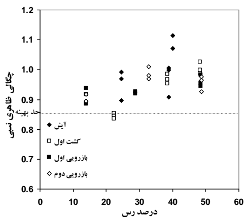
شکل ۲. مقایسه مقادیر چگالی ظاهری نسبی خاک در مزارع نیشکر با حد بهینه RBD برای رشد ریشه گیاه
