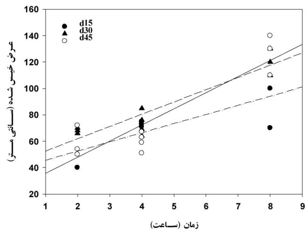
شکل ۱. رابطه بین زمان و عرض خیس شده در عمق (d) ۱۵، ۳۰ و ۴۵ سانتی متر با قطره چکان ۲ لیتر بر ساعت
