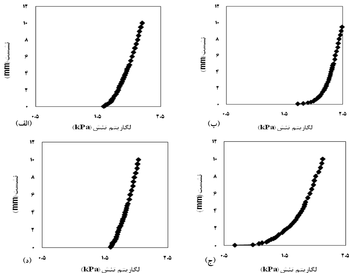
شکل ۲. نمونه‌هایی از نمودار لگاریتم تنش-نشست خاک رس سیلتی در آزمایش نشست صفحه‌ای (PST) بدون بار متراکم‌کننده، الف) رطوبت ۰/۹PL بدون ترخشک شدن، ب) رطوبت ۰/۹PL با ترخشک شدن، ج) رطوبت ۱/۱PL بدون ترخشک شدن و د) رطوبت ۱/۱PL با ترخشک شدن.
