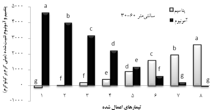
شکل ۴. میانگین پتاسیم و آمونیوم تثبیت شده در اعماق ۰-۳۰ و ۳۰-۶۰ سانتی متری نخلستان آبادان
