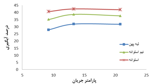
شکل ۸. تغییرات میزان آبیگری سرریزهای جانبی با ارتفاع ۱۲۵ میلی‌متر با باز شدگی ۵ سانتی‌متر در درجه انتهایی
