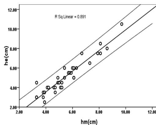
شکل ۸. بررسی آماری و پراکنش داده‌های حاصل از مدل تلاطمی RNG در سطح اطمینان ۹۵٪
