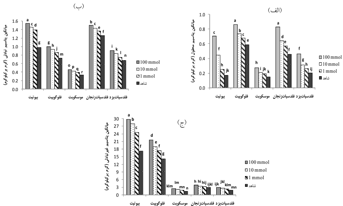
شکل ۱. میانگین پتاسیم محلول (الف)، تبدالی (ب) و غیر تبدالی (ج) آزاد شده تحت تأثیر اسید اگزالیک با غلظت‌های مختلف در کانی‌های بیوتیت، فلوگوپیت، موسکویت، فلدسپات زنجان و فلدسپات یزد (میانگین‌های دارای حرف مشترک در سطح ۵٪ دارای اختلاف معنی‌دار نمی‌باشند)
