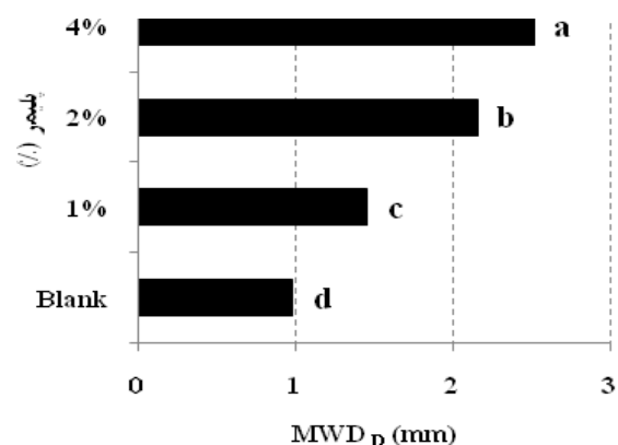
شکل ۹. تأثیر غلظت پلیمر پلی‌اکترولیت آنیونی بر MWDD (میانگین‌های دارای حروف مشابه در سطح ۵ درصد آزمون دانکن فاقد اختلاف معنی دار می‌باشند)
