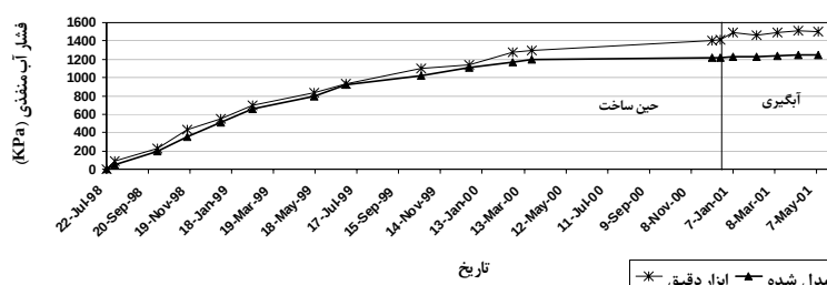
نسبت فشار آب منفذی در مرکز هسته -رقوم ۲۷۰ متر-آبگیری
