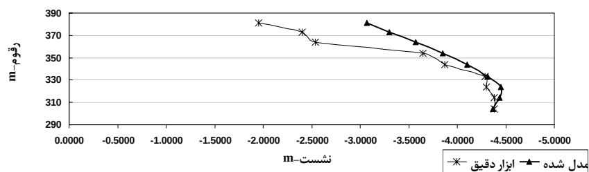
نشست در حالت مخزن نیمه پر تا ۱۳-مه-۲۰۰۱
