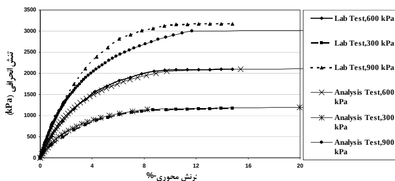
شکل ۵. نتایج کالیبراسیون مصالح هسته سد، M_3 ، با مدل الاستیک غیرخطی و مقایسه نتایج تنش انحرافی- کرنش محوری بین مدل و آزمایشگاه در مصالح هسته در شرایط CD
