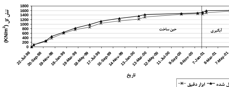
شکل ۱۱. نتایج فشار آب منفذی، نسبت فشار آب منفذی و تنش کل مدل شده و حاصل از ابزار دقیق در ابزار PPE222 و EP2202
