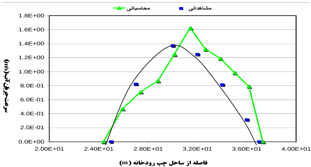
شکل ۷. نمودار تغییرات سرعت آب شبیه‌سازی شده با مدل و اندازه‌گیری شده در مقاطع سه‌گانه
