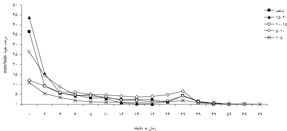
ج) سرعت نفوذ در شدت ترافیک‌های مختلف در مسیر چوبکشی ۱۵-۲۰ سال
