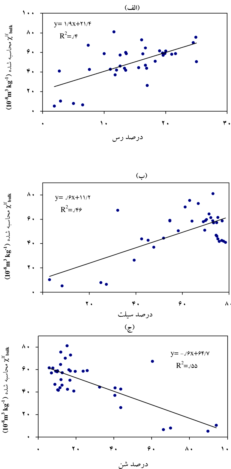
شکل ۳. ارتباط بین \chi_{bulk}^{bf} و (الف) درصد رس، (ب) درصد سیلت و (ج) درصد شن، (نمونه‌های خاک مارنی در نظر گرفته نشده‌اند).
