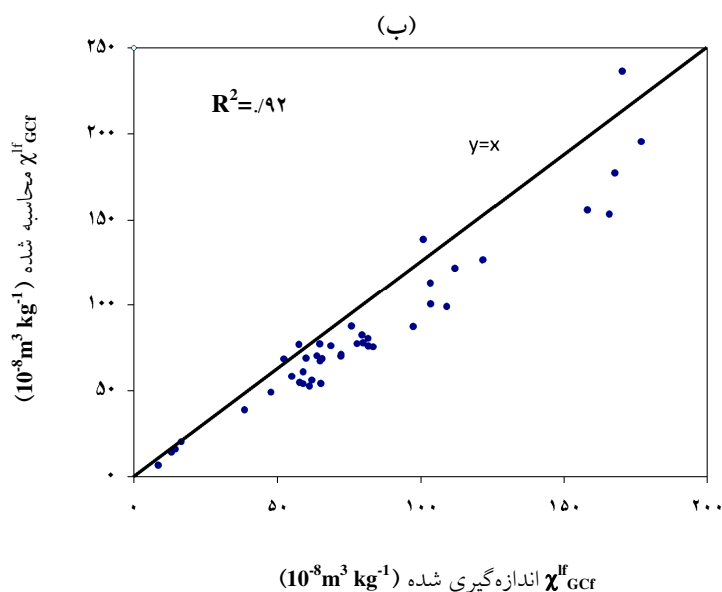
شکل ۲. ارتباط مقادیر اندازه‌گیری شده و محاسبه شده (الف) پذیرفتاری مغناطیسی پس از حذف گچ ( \chi_{Gf}^{lf} ) و (ب) پذیرفتاری مغناطیسی پس از حذف گچ و کربنات‌ها ( \chi_{Gcr}^{lf} )
