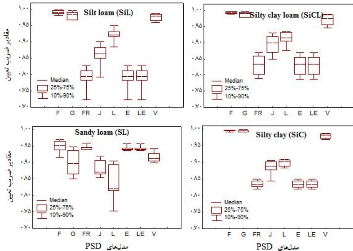
شکل ۴. نمودارهای جعبه‌ای ضرایب تعیین هشت مدل PSD مورد مطالعه در چهار کلاس بافت SiC، SiCL، SiL و SL. مدل = F) مدل فردلاند، G = مدل گمپرتز، FR = مدل فراکتال، J = مدل جیکی، L = مدل لگاریتمی، E = مدل نمایی، LE = مدل لگاریتمی-نمایی و V = مدل ون گنوختن)
