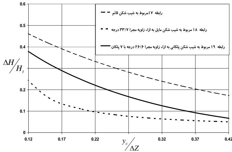
شکل ۱۰. مقایسه استهلاك انرژی نسبی بر اساس روابط پیشنهادی جدول ۲ در ۳ تیپ مختلف شیب شکن
