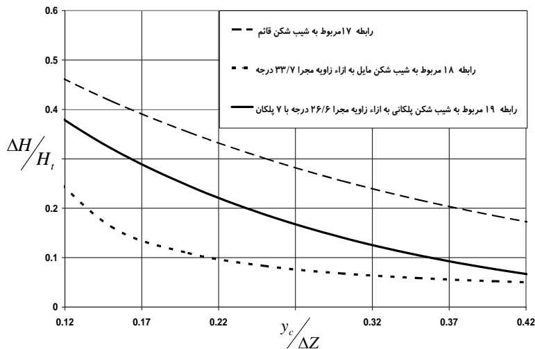
شکل ۱. مقایسه استهلاک انرژی نسبی بر اساس روابط پیشنهادی جدول ۲ در ۳ تیپ مختلف شیب شکن
