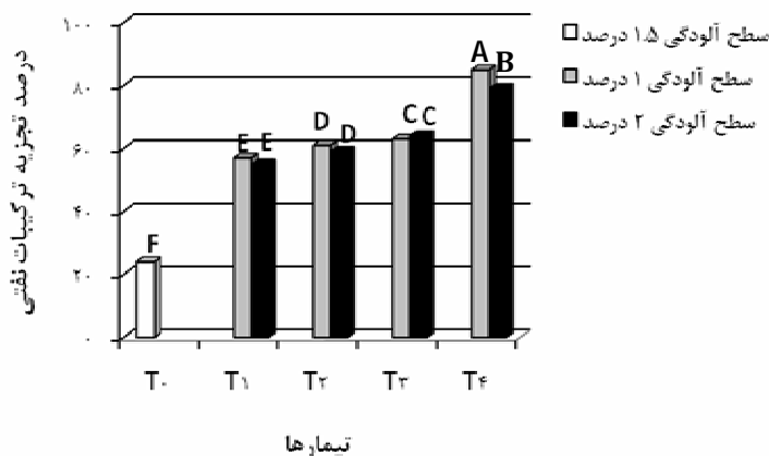
شکل ۱. راندمان تیمارهای T 0 : تیمار شاهد T 1 : تیمار کشت شبدر با مایه زنی میکوریزا T 2 : کشت شبدر با مایه زنی میکوریزا T 3 : کشت شبدر با مایه زنی باکتری‌های تجزیه‌گر T 4 : کشت شبدر با مایه زنی میکوریزا و باکتری‌های تجزیه‌گر برای تجزیه هیدروکربن‌های نفتی در سطوح مختلف آلودگی
