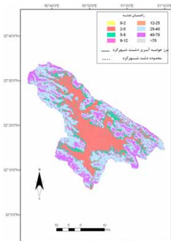
شکل ۶. نقشه شیب در حوضه آبریز دشت شهرکرد
