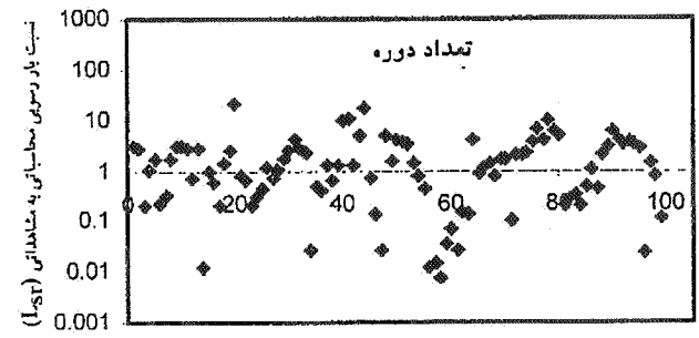
نمودار ۳-۳. روش ساماگا، رودخانه کارون
