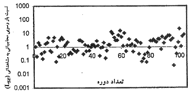
نمودار ۱-۳. روش ساماگا، رودخانه دز
