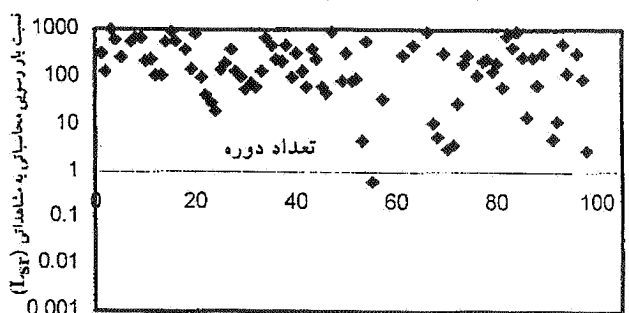
نمودار ۱۰-۳. روش فاضل، رودخانه کارون
