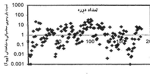
نمودار ۴-۴. روش توفالتی، رودخانه مارون
