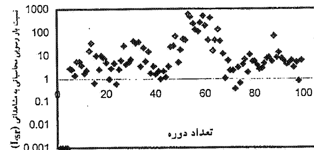
نمودار ۸-۱. روش یانگ، رودخانه دز
