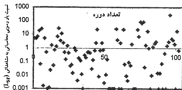
نمودار ۵-۱. روش وان ریجن، رودخانه دز
