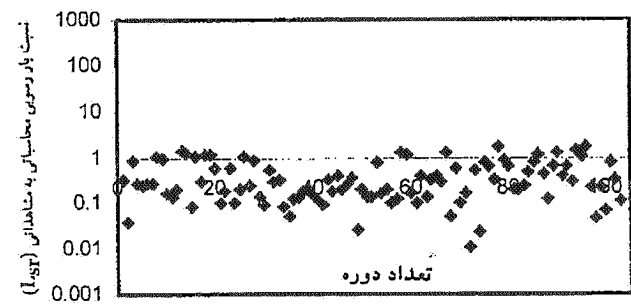
نمودار ۱-۴. روش توفالتی، رودخانه دز
