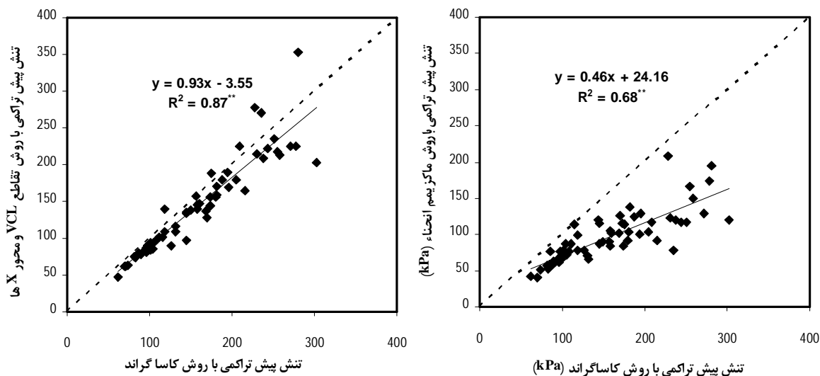
شکل ۶. مقایسه مقادیر تنش پیش تراکمی تعیین شده توسط روش‌های نقطه بیشینه انحناء و تقاطع خط فشردگی بکر با محور Xها با روش کاساگراند در آزمایش PST.
