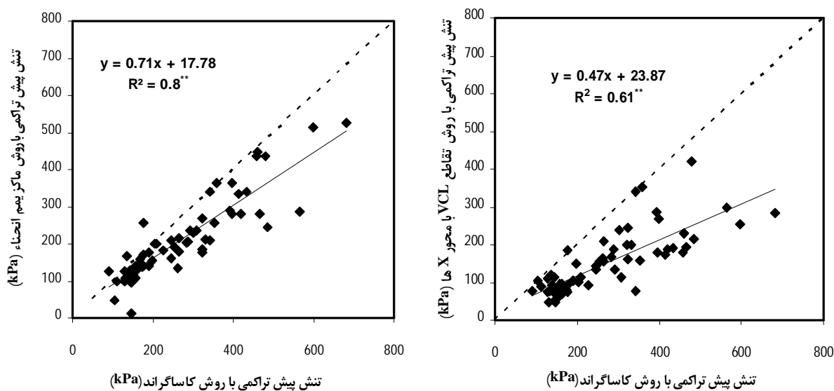
شکل ۶. مقایسه مقادیر تنش پیش تراکمی تعیین شده توسط روش‌های نقطه بیشینه انحناء و تقاطع خط فشردگی بکر با محور Xها با روش کاساگراند در آزمایش PST.
