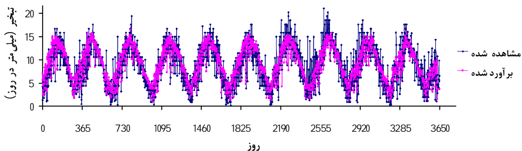
شکل ۵. تغییرات زمانی مقادیر تبخیر از تشت مشاهده شده و برآورد شده، بر اساس ترکیب شماره ۵ در دوره آماری (۱۳۷۵ الی ۱۳۸۴)
